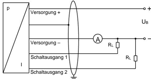
2-Leiter-System (Strom)
