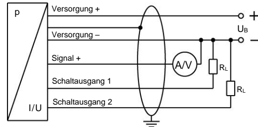
3-Leiter-System (Strom/Spannung)
